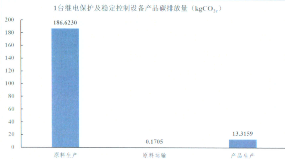
图 2 1 台继电保护及稳定控制设备产品各阶段碳足迹排放量
