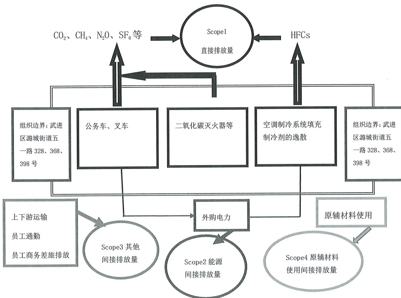
图 2 排放源示意图
